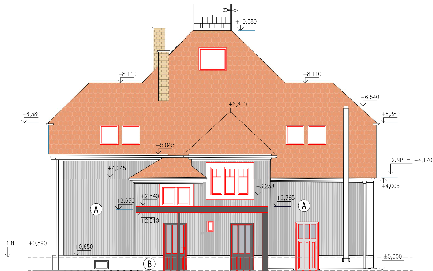
POHLED SZ
