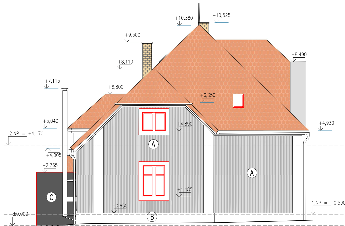
POHLED SV doupravit
